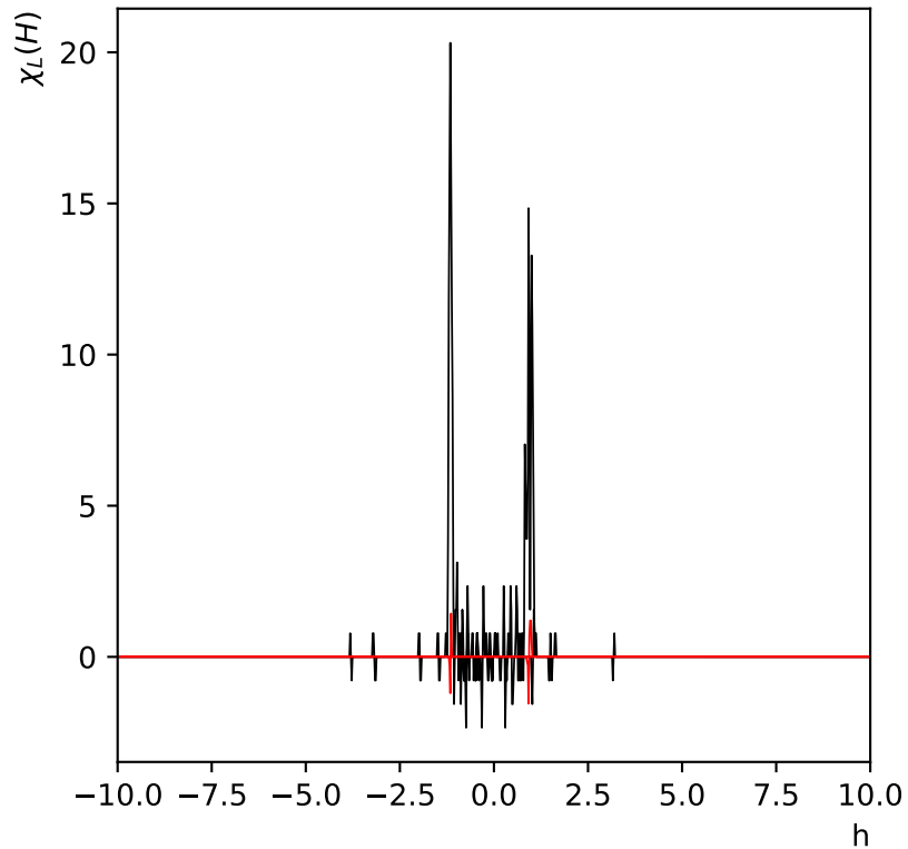
\chi_L(H) réseau de taille L=8 à T=1.5
