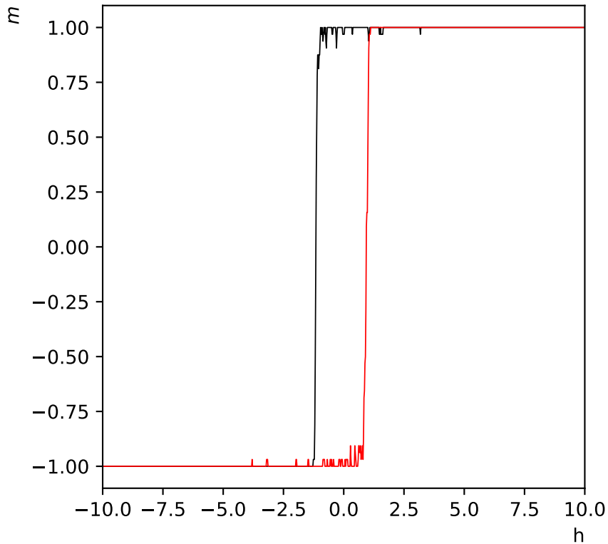
Hystérésis de l'aimantation réseau de taille L=8 - h=10 à T=1.5
